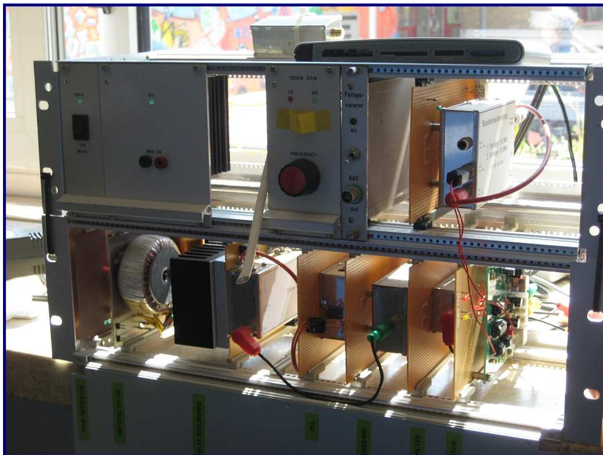
Abbildung 5: 23cm – ATV-Sender (nicht zu sehen: Die 50W-PA von DG0VE)
